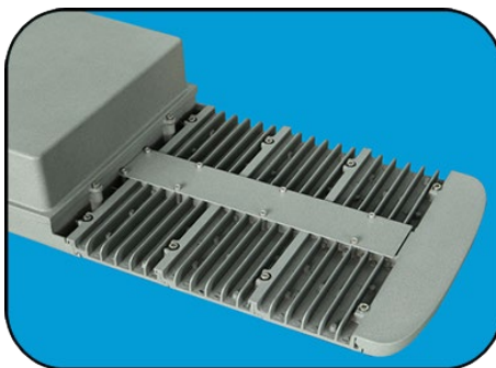
高导热压铸铝合金散热模组
