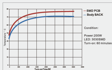
升温曲线
