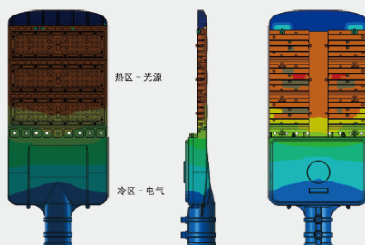
传导散热示意图
